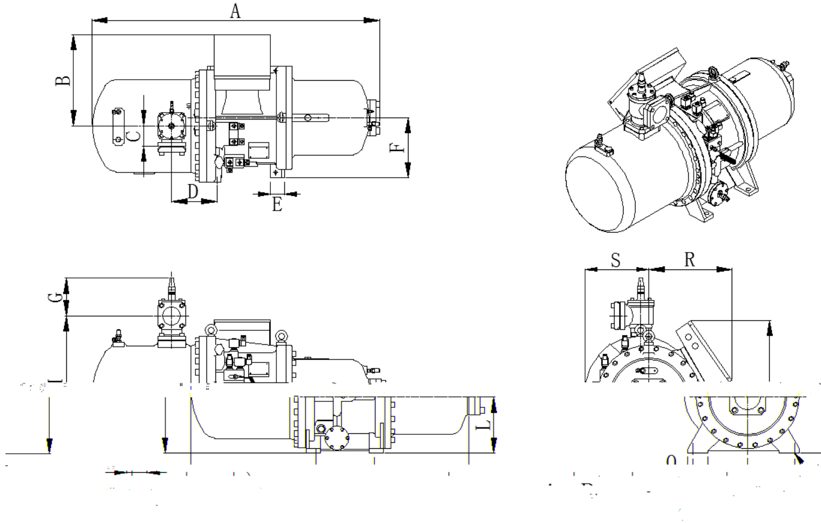
RC2-300E~930E 标准油分外观尺寸图
